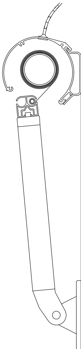
Lodret snit af kasse med bundprofil
