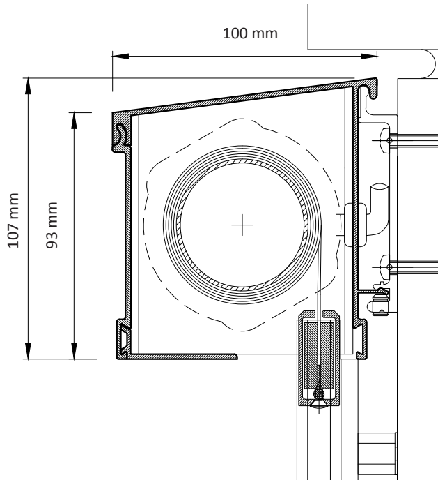
Lodret snit af kasse med bundprofil, 1:2
