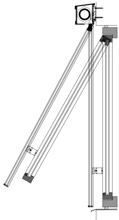
El-betjent på mur med glidebeslag
