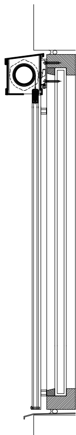
El-betjent på fast vindue
