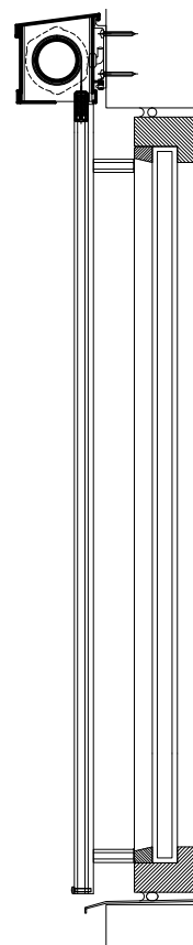
El-betjent på mur ved fast vindue
