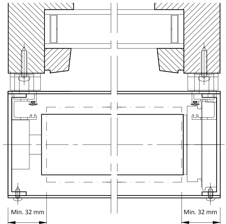
Vandret snit af kasse, 1:2
